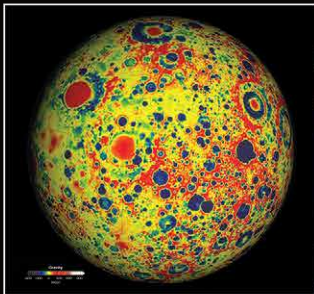
MOON GRAVITY MAP
